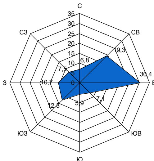
Рисунок 1.1-1. Роза ветров
